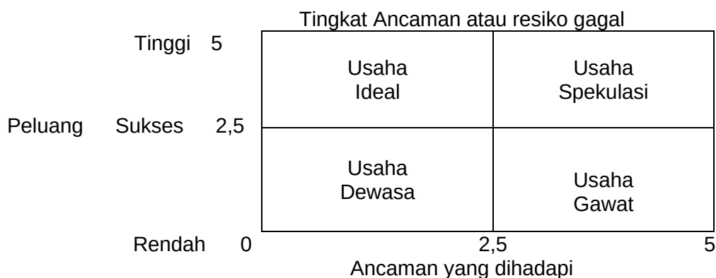
Gambar 1 . Matriks ETOP
