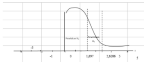
Gambar 2. Kurva Uji t
