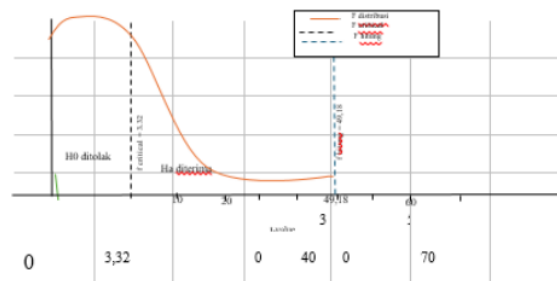
Gambar 4 Kurva Uji f
