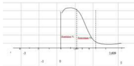
Gambar 3 Kurva Uji t
